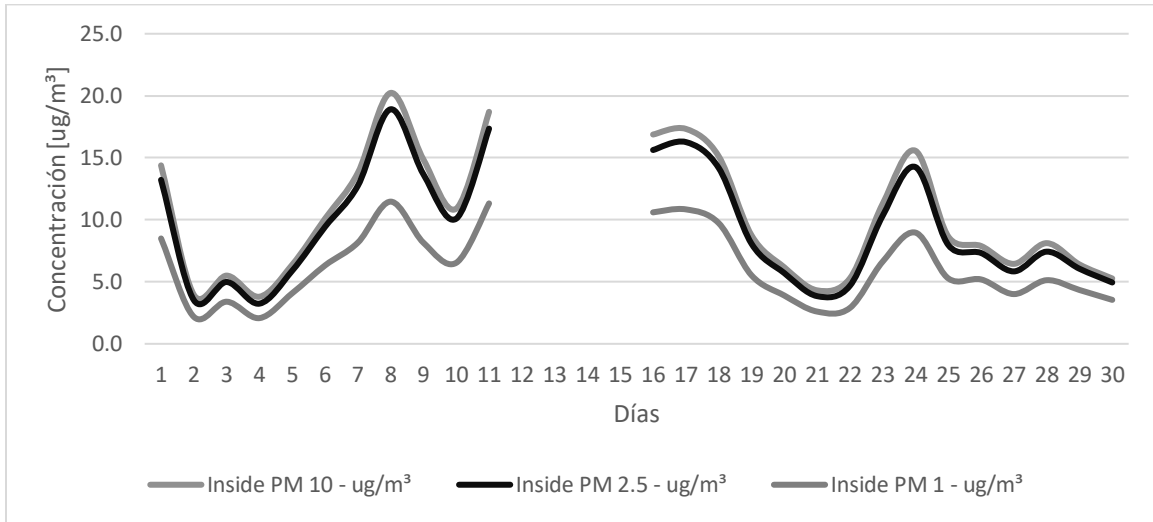
Figura 7. Concentración de partículas
