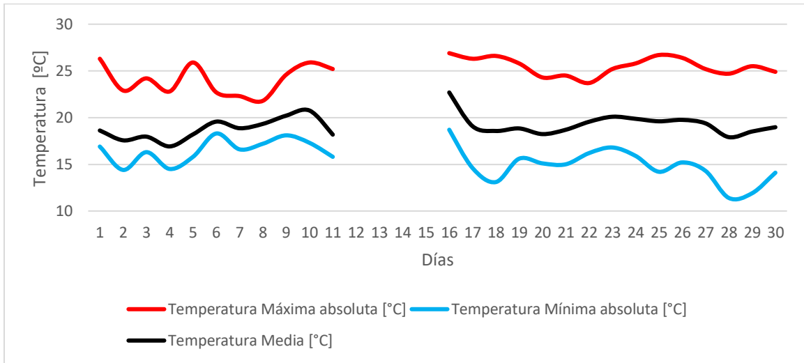
Figura 2. Temperatura del aire diaria (media, máxima y mínima). Enero de 2022
