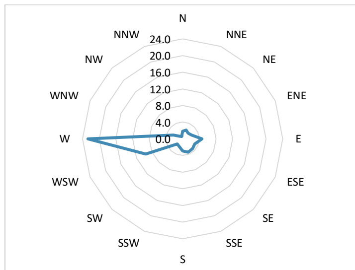
Figura 3. Dirección desde donde provienen los vientos. Enero de 2022
