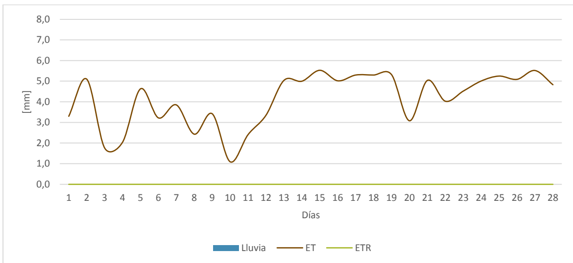
Figura 6. Relación entre las variables del balance hídrico
