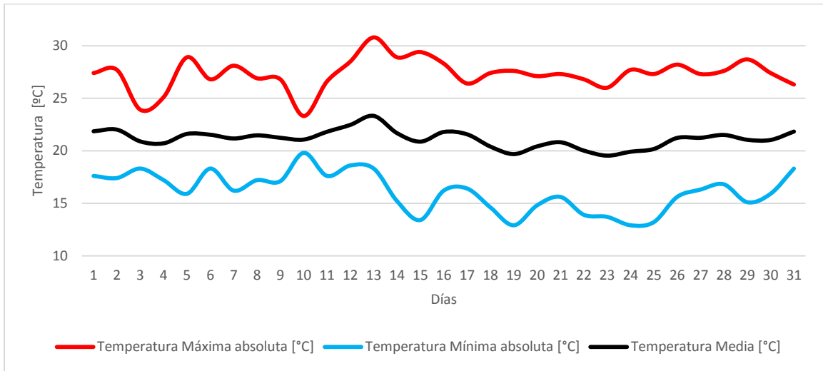
Figura 2. Temperatura del aire diaria (media, máxima y mínima). Marzo de 2022
