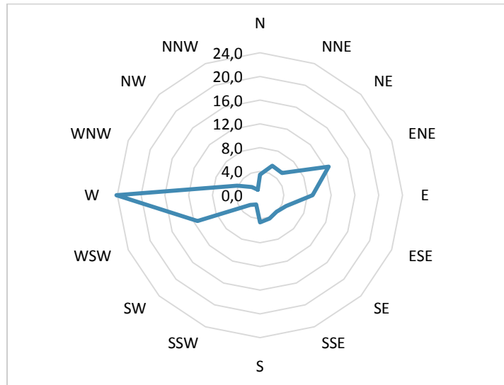
Figura 3. Dirección desde donde provienen los vientos. Marzo de 2022
