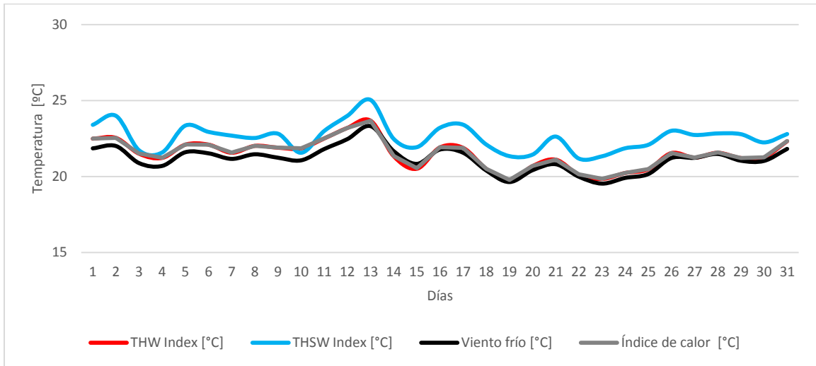
Figura 7. Índices de confort térmico. Marzo de 2022
