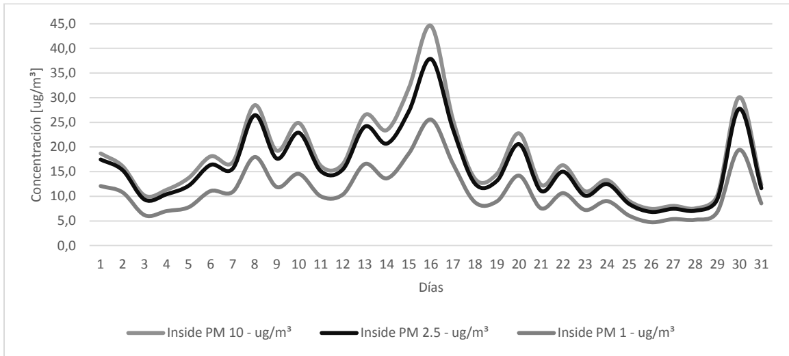
Figura 8. Concentración de partículas
