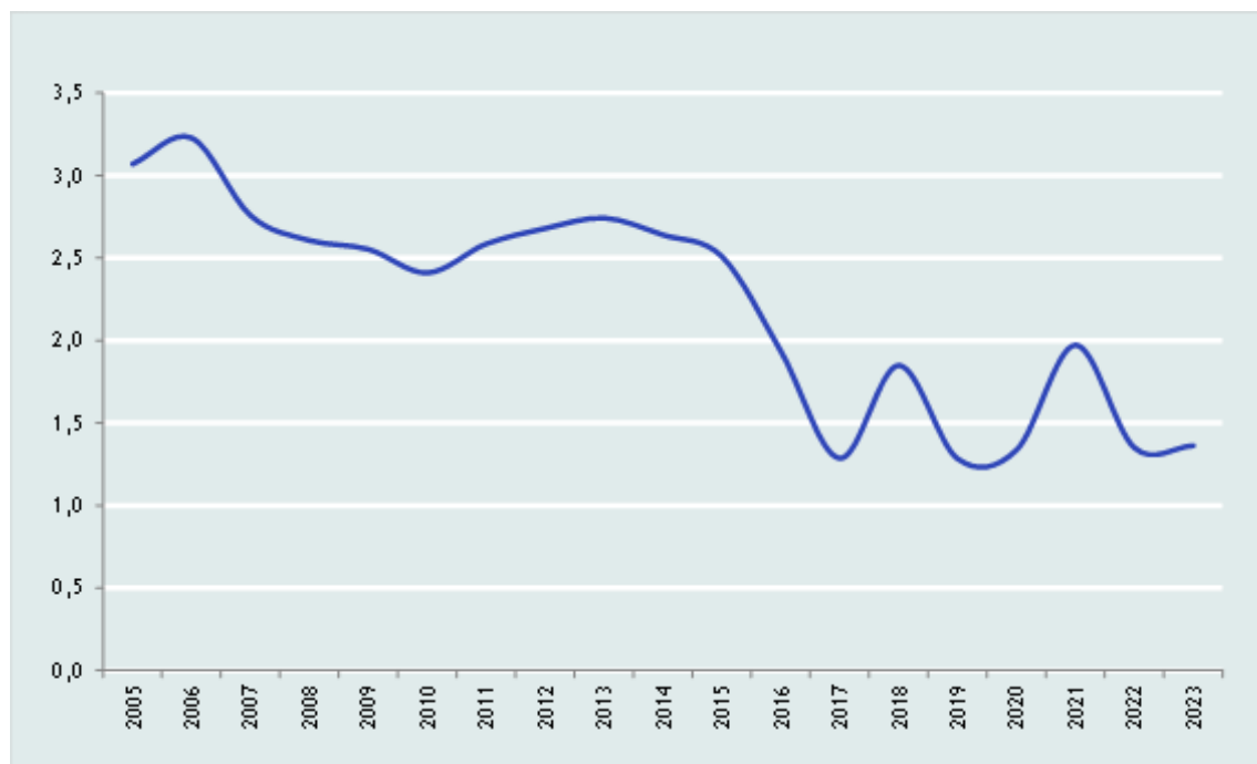
Gráfico 19: Multiplicador monetario
