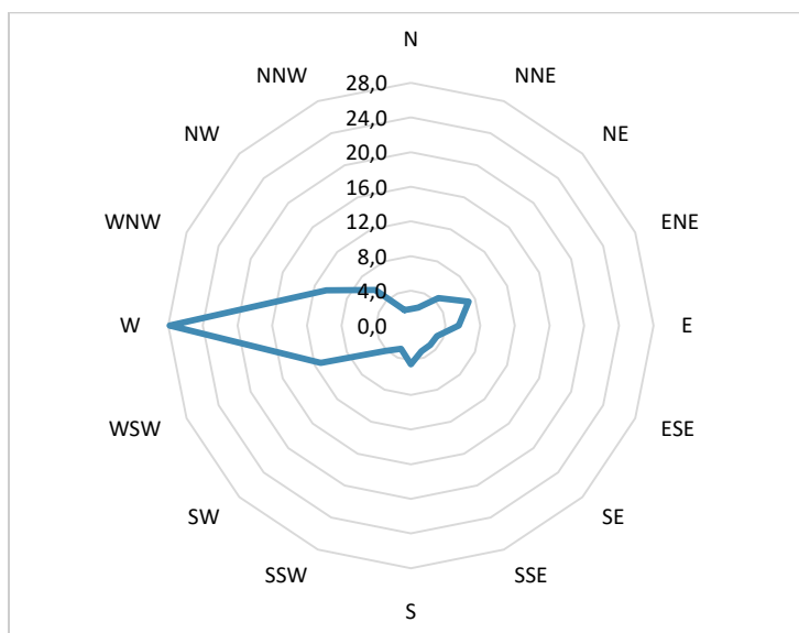
Figura 3. Dirección desde donde provienen los vientos. Agosto de 2023
