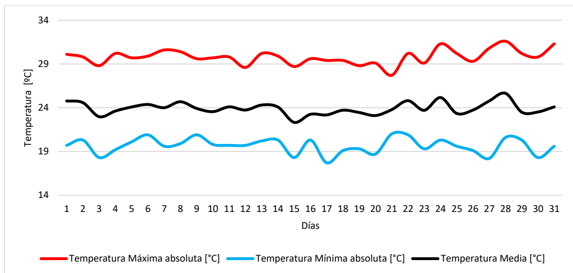
Figura 2. Temperatura del aire diaria (media, máxima y mínima). Agosto de 2023
