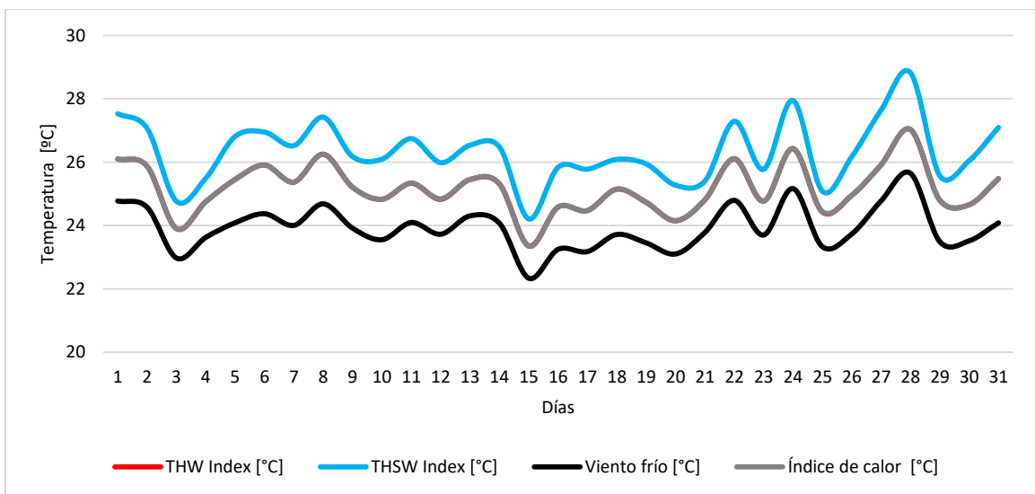
Figura 7. Índices de confort térmico. Agosto de 2023
