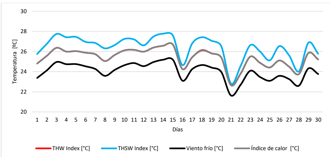
Figura 7. Índices de confort térmico. Septiembre de 2023
