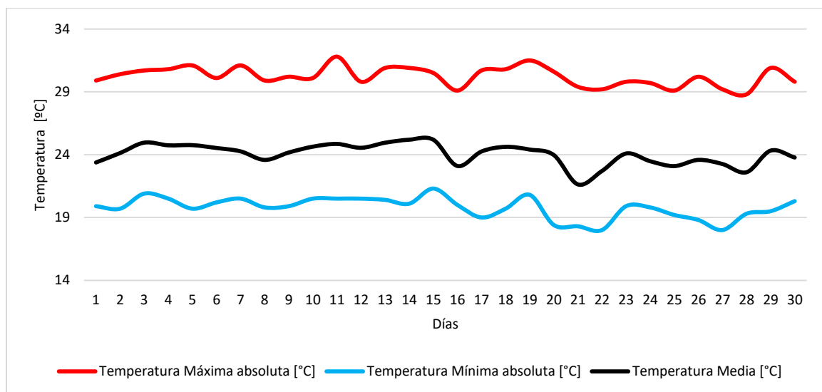
Figura 2. Temperatura del aire diaria (media, máxima y mínima). Septiembre de 2023
