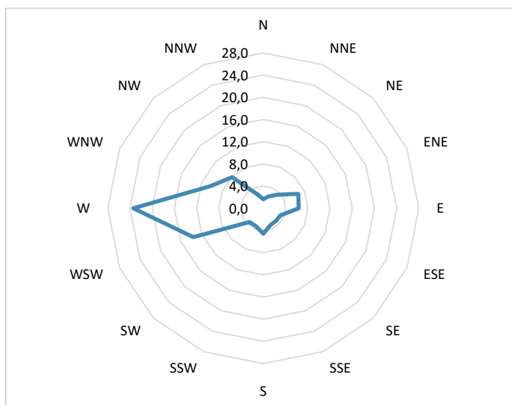
Figura 3. Dirección desde donde provienen los vientos. Septiembre de 2023
