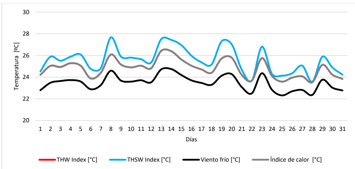
Figura 7. Índices de confort térmico. Octubre de 2023
