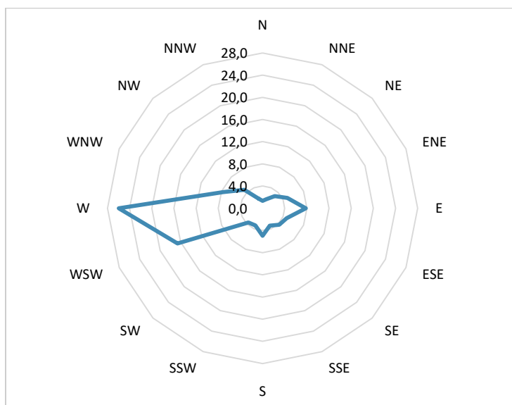
Figura 3. Dirección desde donde provienen los vientos. Octubre de 2023
