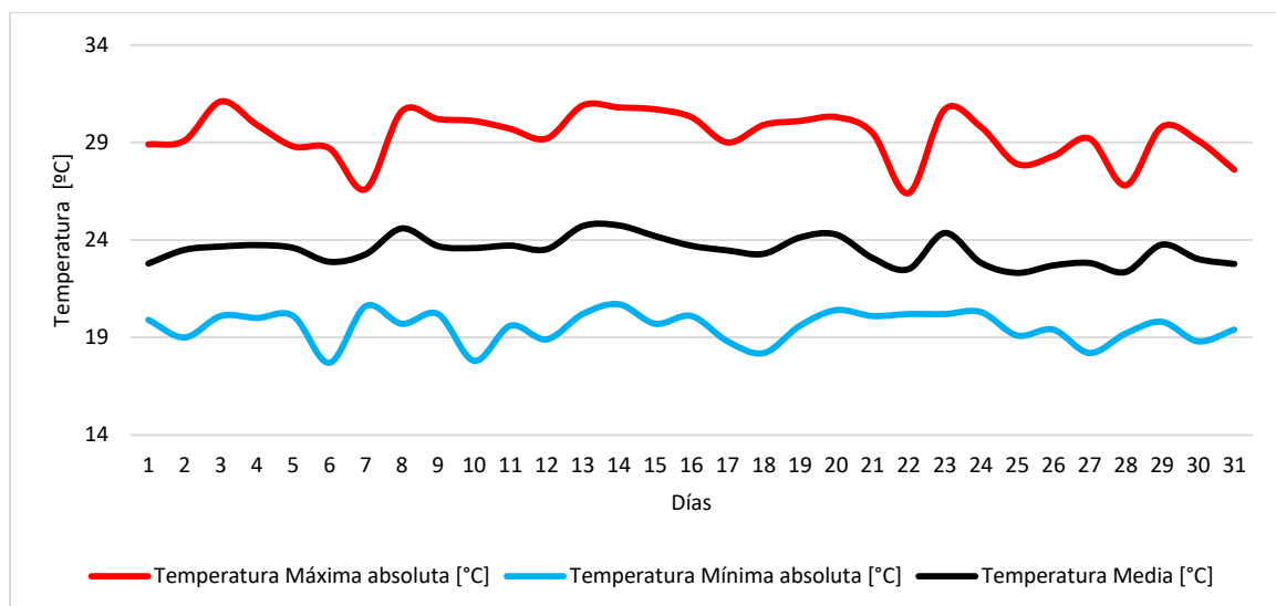
Figura 2. Temperatura del aire diaria (media, máxima y mínima). Octubre de 2023
