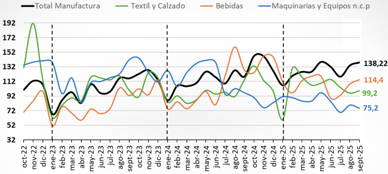
Figura 3.3: Peores desempeños (1)
