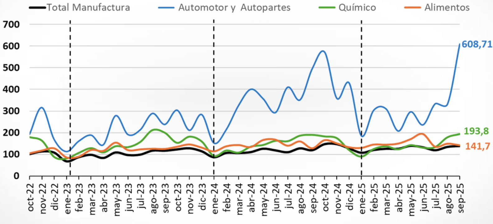
Figura 3.2: Mejores desempeños (2)
