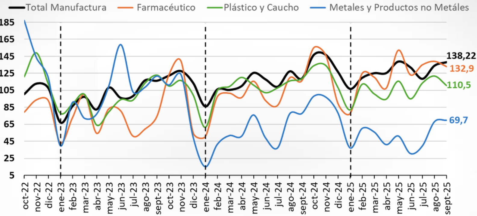
Figura 3.4: Peores desempeños (2)
