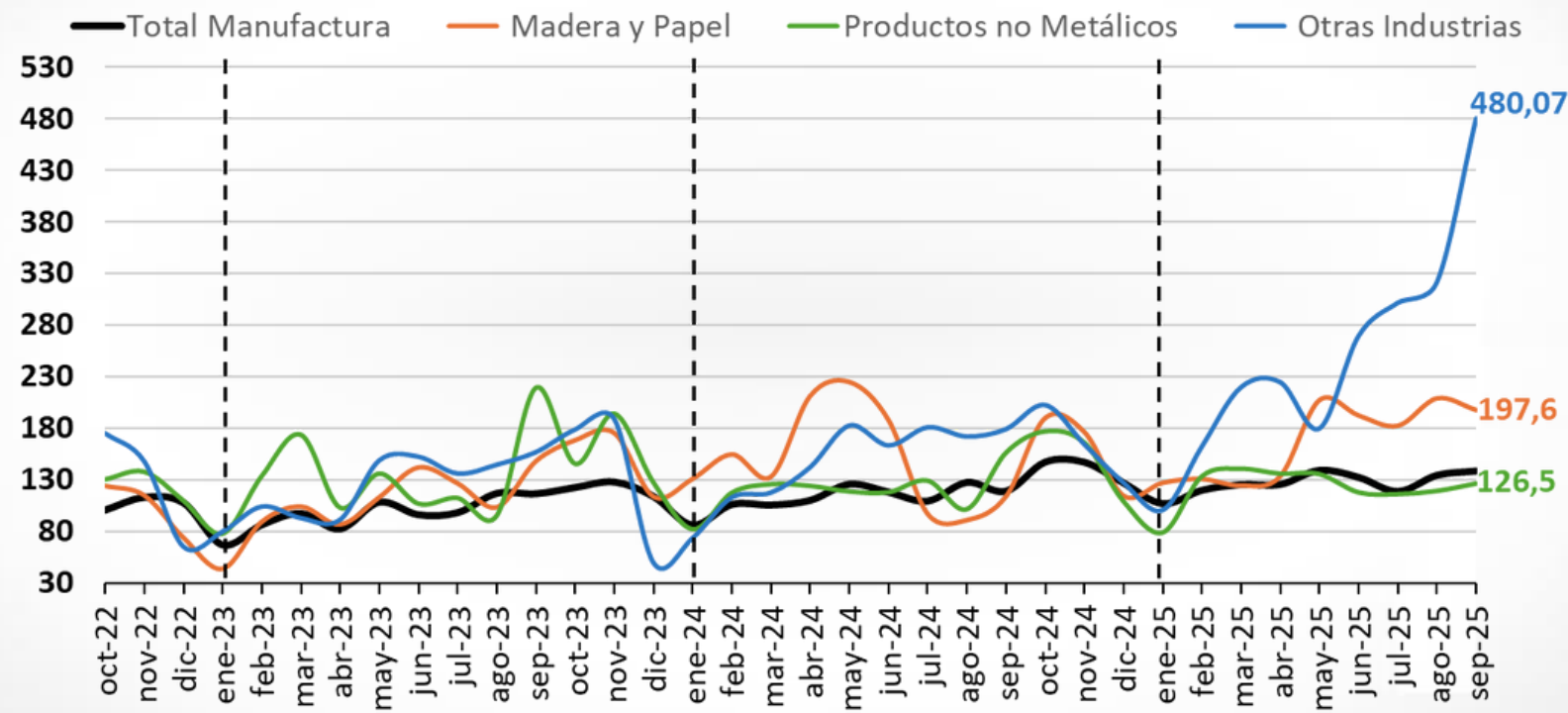
Figura 3.1: Mejores desempeños (1)
