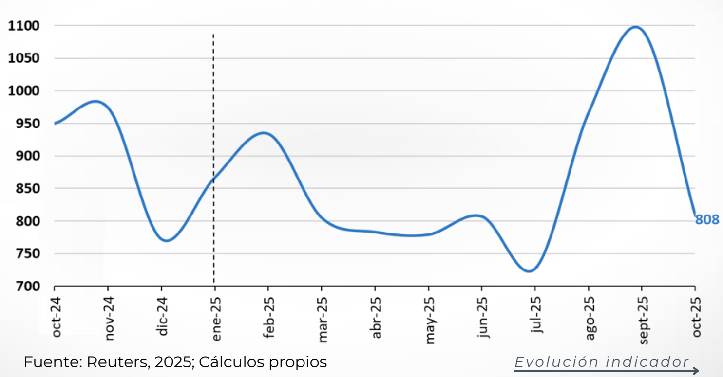
Figura 2.6: Exportaciones petroleras de Venezuela (promedio mensual, mbd)
