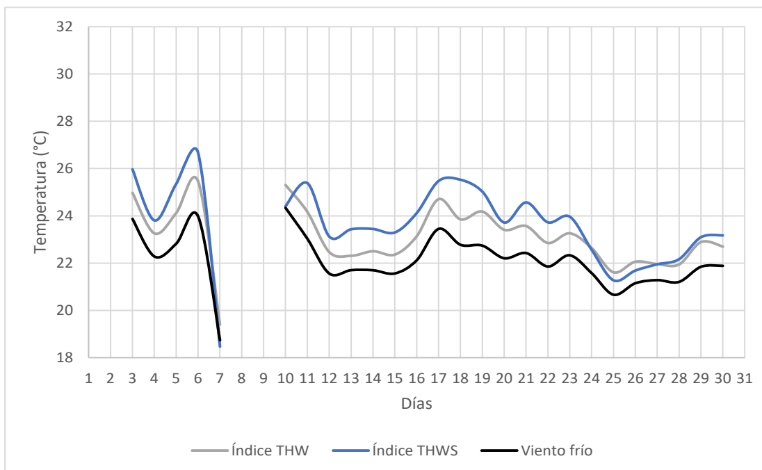
Figura 7. Índices de confort térmico
