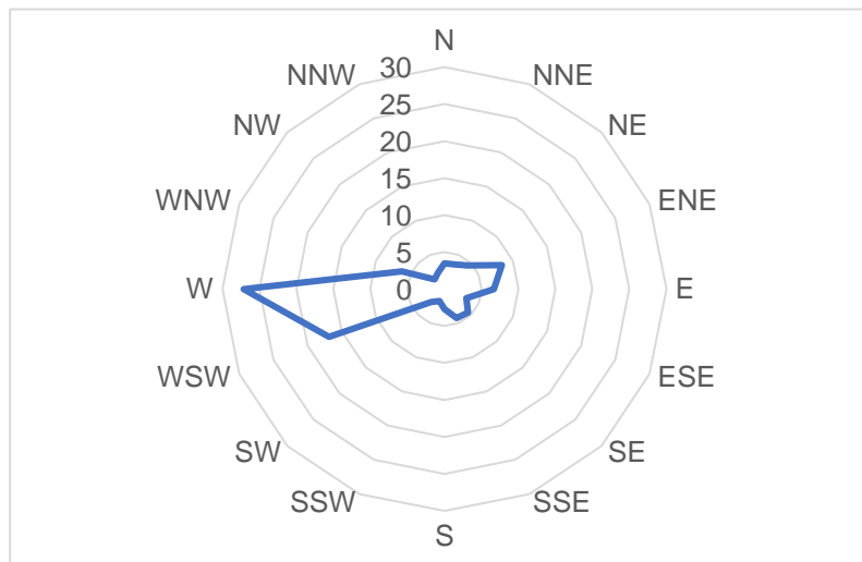
Figura 3. Dirección de los vientos
