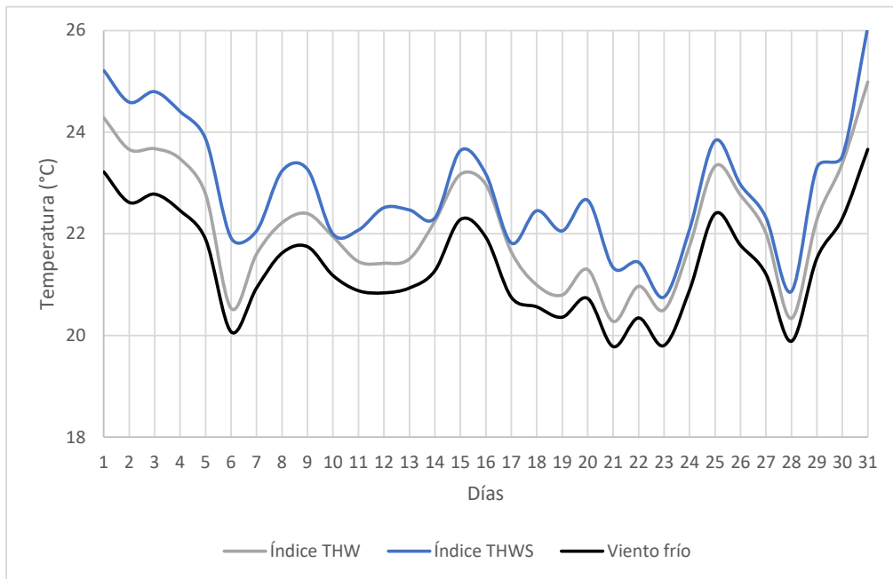
Figura 7. Índices de confort térmico
